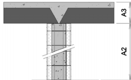
Figure 37 Avec dalle autoportant et couche de pression en béton
