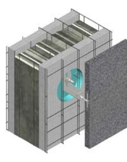
Figure 45 Ancres mécaniques pour la pierre naturelle ou le revêtement
