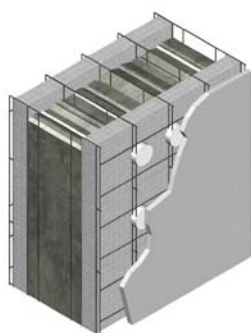
Figure 43 Panneau de finition collé par plots
