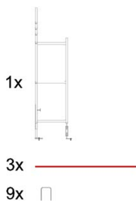
Figure 21 1 set étais = 1 étais, 3 lattes, 9 profils en U
