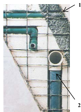
Figure 30 Conduits intégrés dans le béton et l'isolation, 1 avant le coulage du béton 2 dans l'isolation (couper ou faire fondre)
