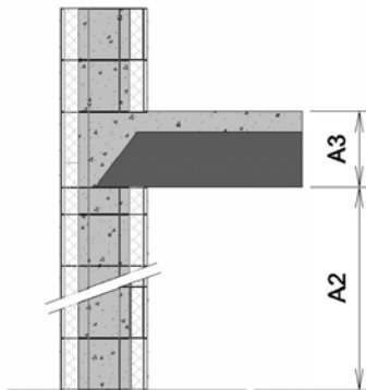
Figure 36 Avec dalle autoportant et couche de pression en béton
