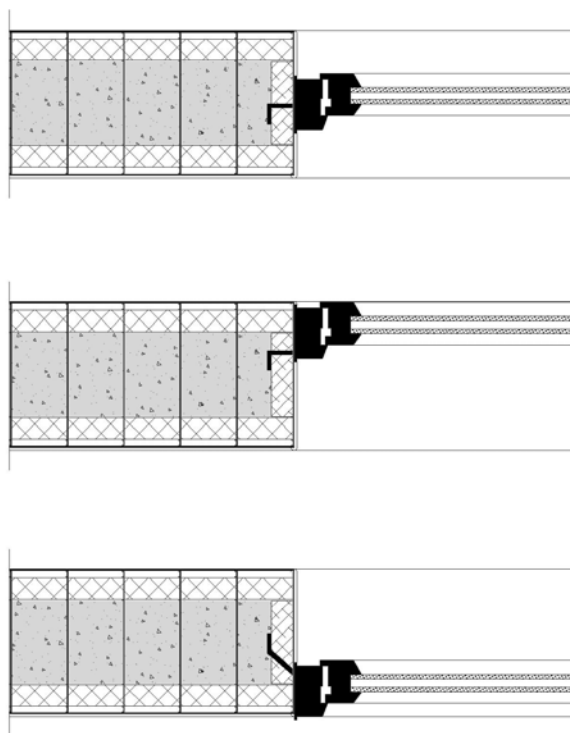
Figure 32 Coupe horizontale : fenêtre dans l'épaisseur, à l'intérieur et à l'extérieur du mur
