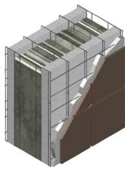
Figure 44 Carrelage sur un base de ciment
