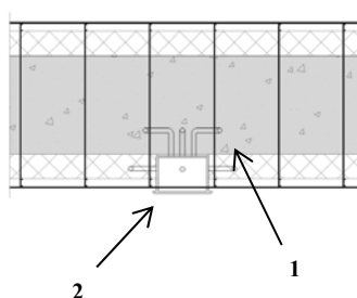
Figure 30 Conduits intégrés dans le béton et l'isolation, 1 avant le coulage du béton 2 dans l'isolation (couper ou faire fondre)
