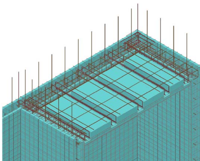
Figure 82 Renforcement d'une dalle
