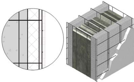
Figure 40 Avec treillis d'accrochage de 1 cm (double fils), enduit de \pm 20 mm
