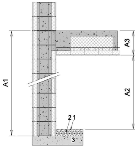
Figure 34 Avec module dalle SISMO®
