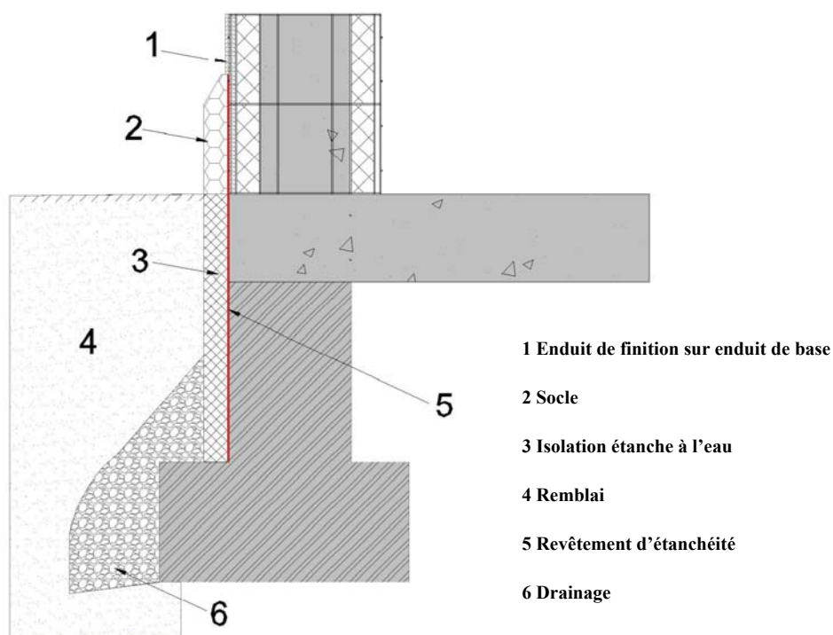
Figure 39 Finition d'un soubassement traditionnel
