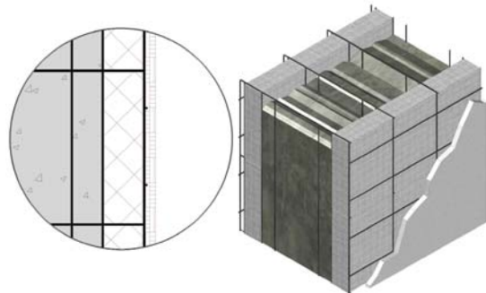
Figure 41 Sans treillis d'accroche (simple fils), enduit de \pm 10 mm
