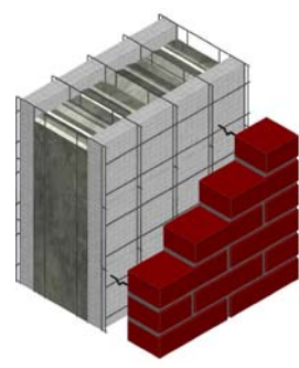
Figure 46 Façade de briques avec fixation mécanique
