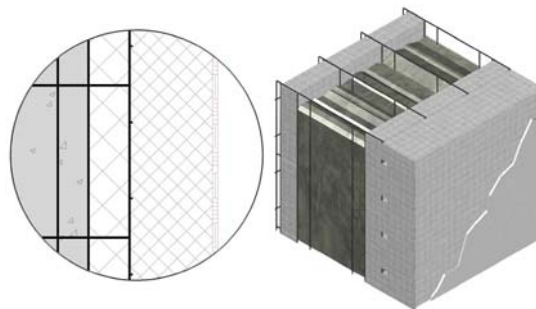
Figure 42 Sur un panneau Plus , enduit de \pm 5 mm
