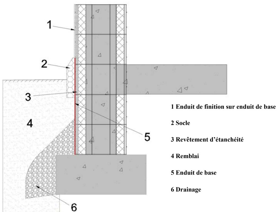
Figure 38 Finition d'un soubassement SISMO®
